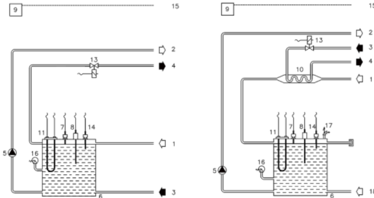
Refrigeración directa
